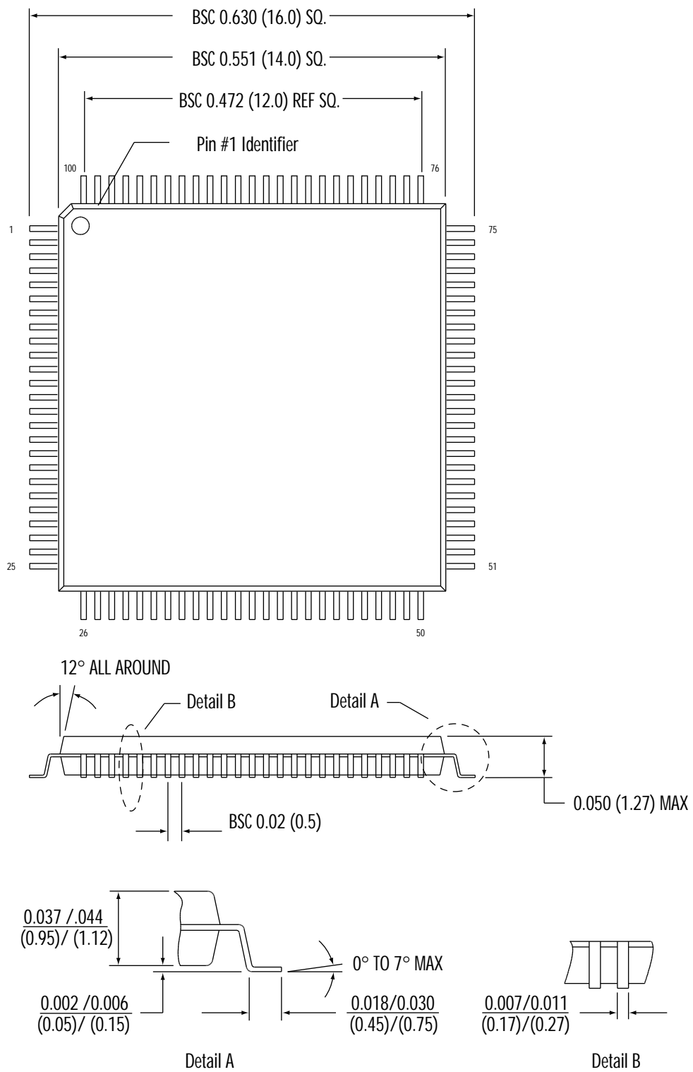
Figure 47. Q1900 VTQFP Package Diagram
